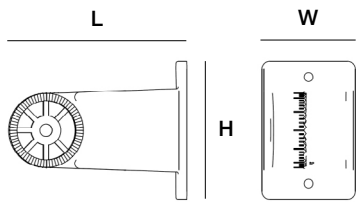
SL (Square Pole L)
